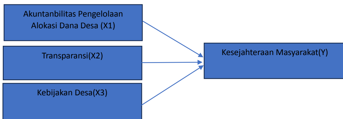
Gambar 1. Kerangka Bepikir
